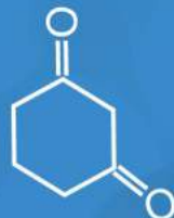
1,3-CYCLOHEXANEDIONE
