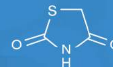
2,4-THIAZOLIDINEDIONE
